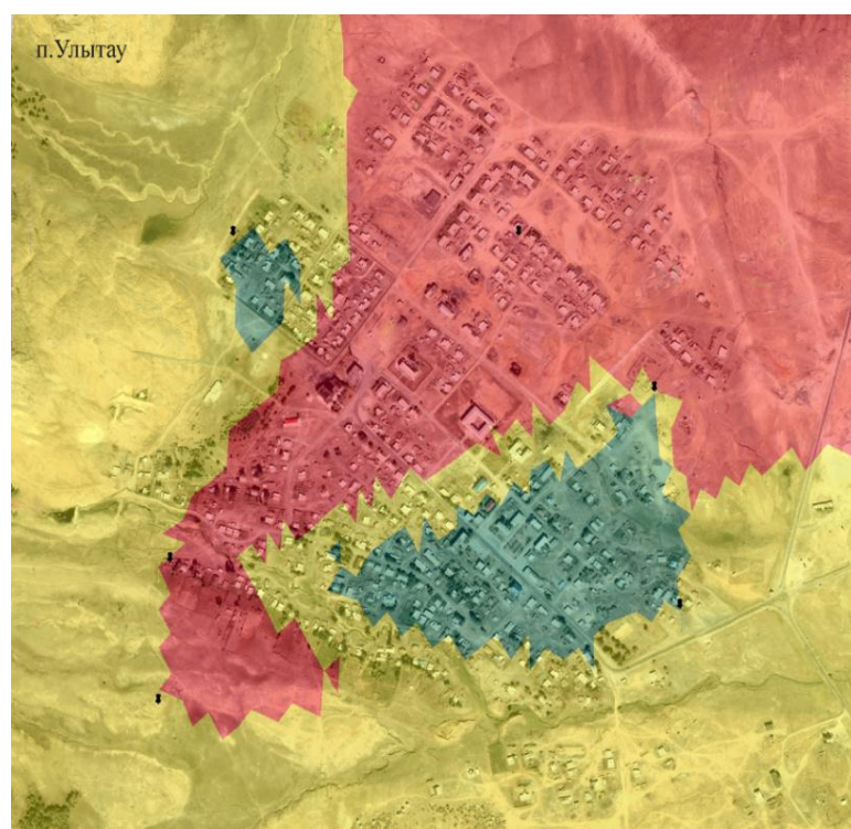
Рисунок 3. Содержание естественного радионуклида ^{226}\text{Ra} в почве п. Улытау
