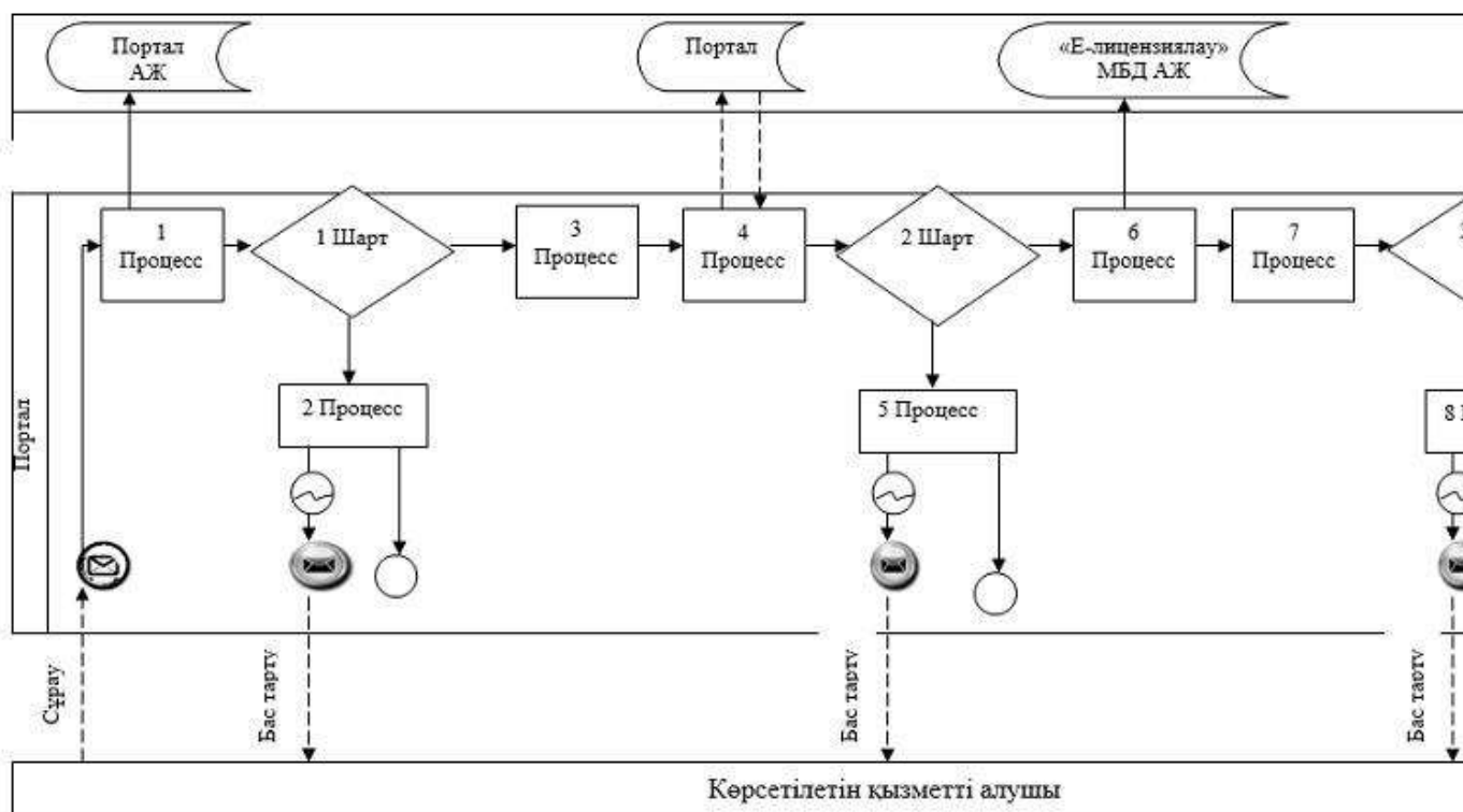
Портал арқылы мемлекеттік қызметті көрсетуге тартылған ақпараттық жүйелердің өзара функционалдық іс-қимылының диаграммасы
