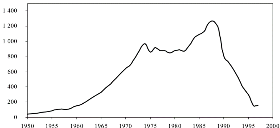
Сурет 3. Әлемде озонды бұзатын заттар өндірісі 1950ж.-1997ж.
