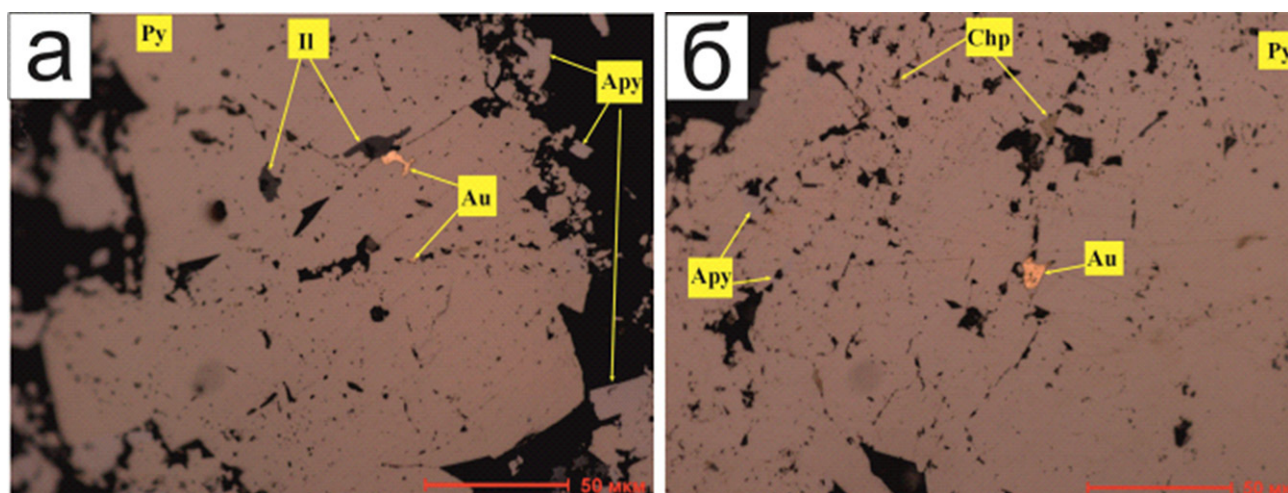
а – микровключения золота (Au) и ильменита (Il) в пирите (Py); б – микровключения золота (Au), арсенопирита (Apy) и халькопирита (Chp) в пирите (Py)
