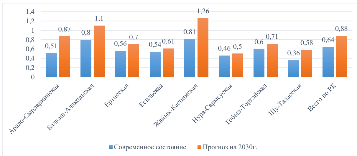
Рис. 3 – Динамика экологического спроса природно-хозяйственных систем на водные ресурсы (доля от нормы стока, б.р.)
