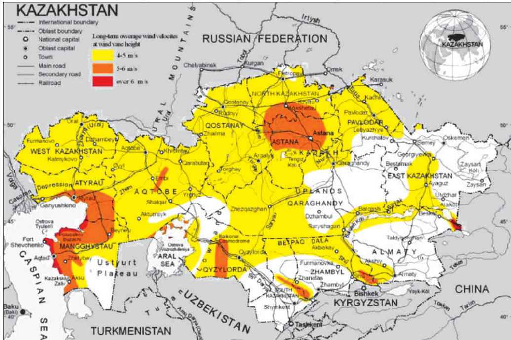
Рисунок 5 – Карта ветров (ветровой атлас) Казахстана с перспективными для строительства ВЭС регионов
